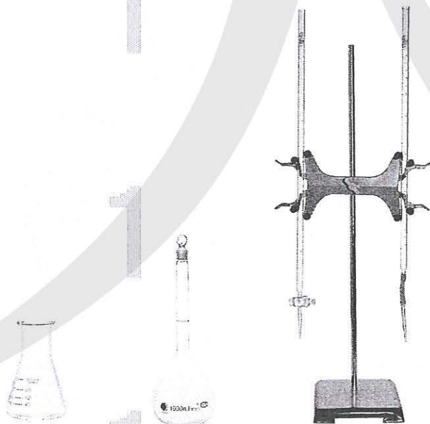
图3-10 酸碱中和滴定常用的仪器
