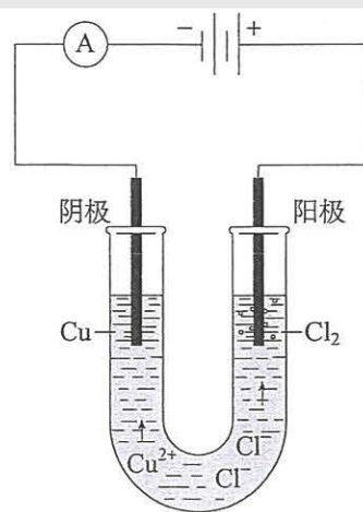
图4-9 氯化铜溶液的电解装置示意图
