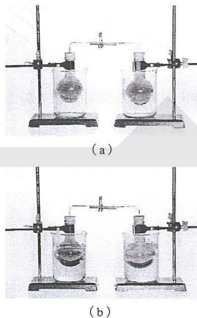
图2-7 装有 \text{NO}_2 和 \text{N}_2\text{O}_4 的烧瓶（a），分别浸泡在热水（左）和冰水（右）中（b）
