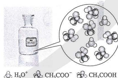
图3-2 CH 3 COOH在水中电离示意图
