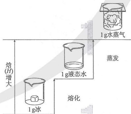
图 1-6 水的聚集状态变化时的焓变
